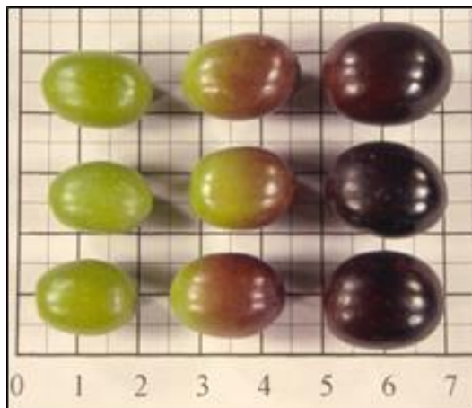
Figura 1: Esempio di invaiatura su cv. Leccino, varietà caratterizzata da una maturazione precoce
